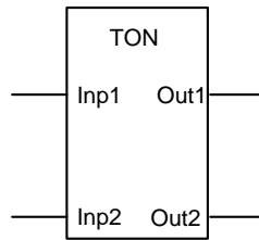
5.2. ábra. A TON szabványos funkció blokkja két bemeneti és két kimeneti paraméterrel.
