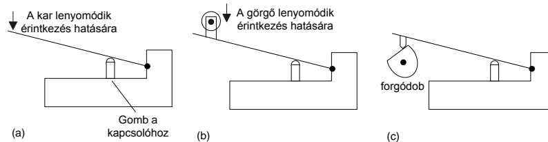
3.24. ábra. – : Végállás kapcsolók.
