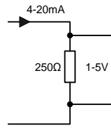
3.18. ábra. – : Szabványos analóg jelátalakítás.
