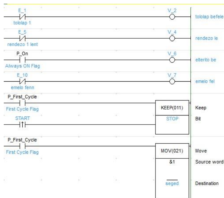
9.17.b ábra – : A kezdobeállítások, LAD nyelven írt akció.
