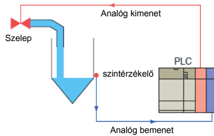
3.16. ábra. – : Tipikus analóg I/O rendszer.
