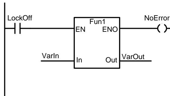
5.6. példa. – : A függvény grafikus jelölése az EN/ENO paraméterekkel a LAD nyelvben.
